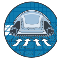
Filtration
