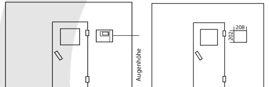
Wandausschnitt bei Montage in der Wand
